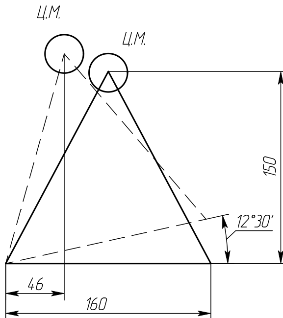
Рисунок 1- Схема устойчивости электронасосного агрегата типа ВКС1/16.
