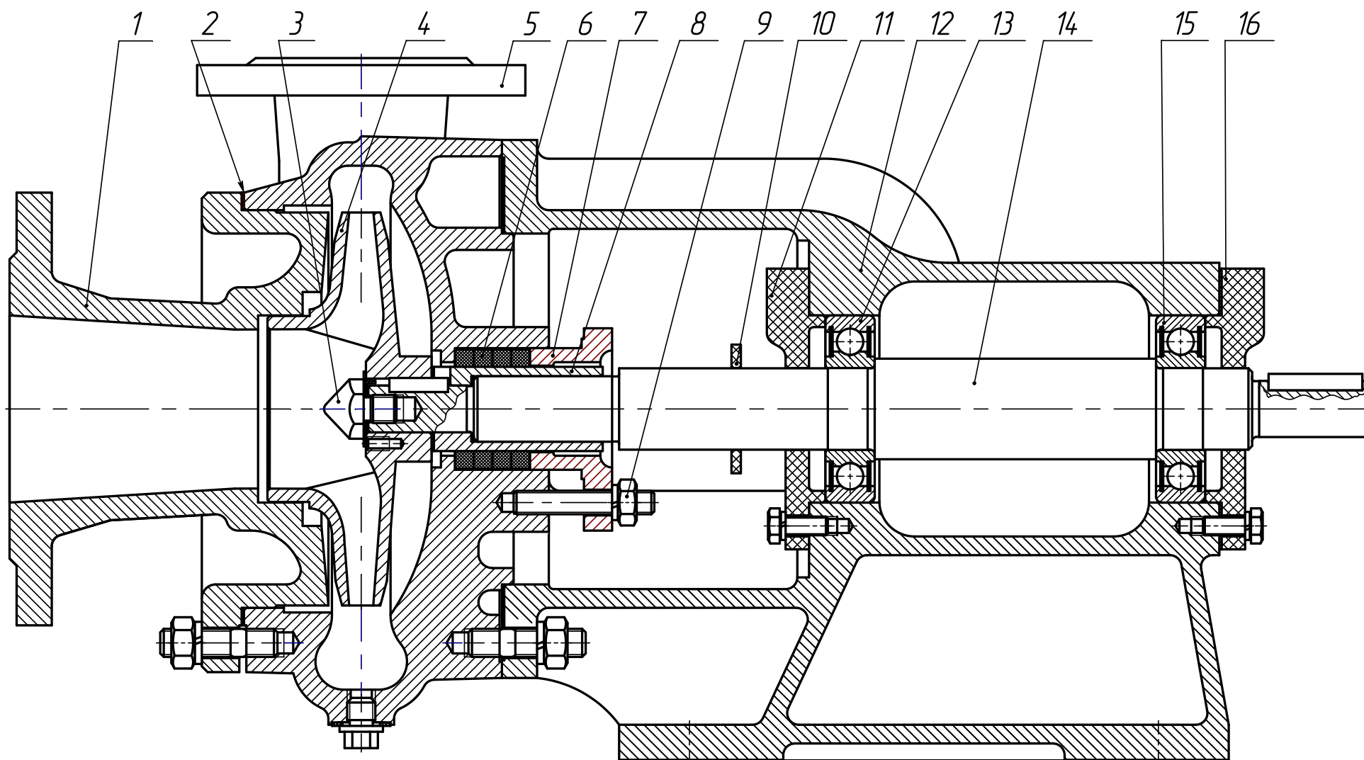
Рисунок 1 - Разрез насоса
